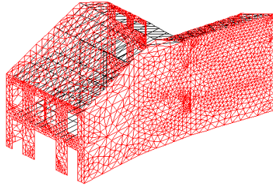
Fig. 5 - A Modelling
