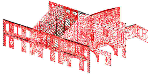
Fig. 6 - B Modelling
